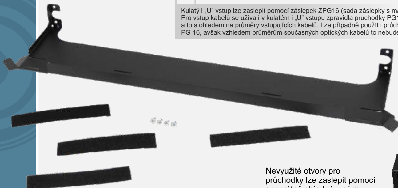
Pořadač patchcordů pro rozváděč SLIDE
