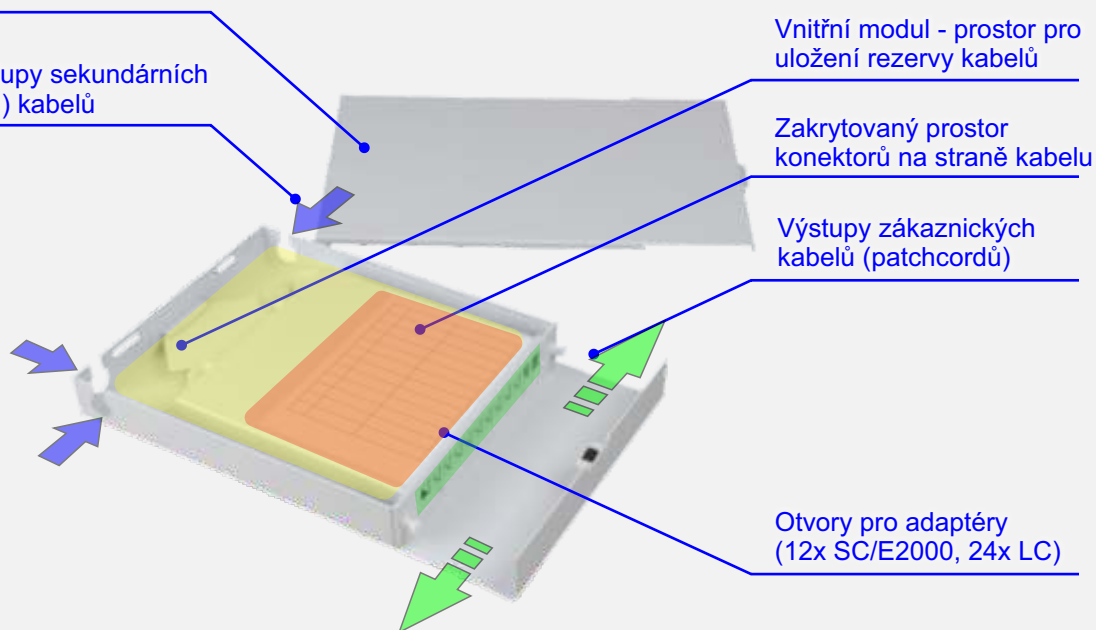
Skladba rozváděče
