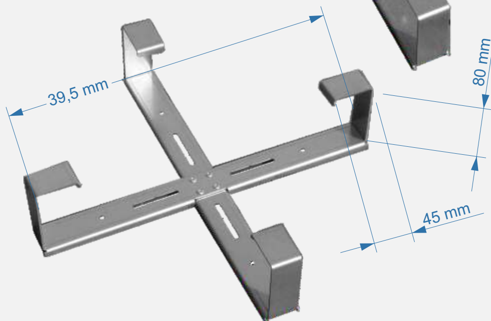
704 000 000 - Kříž kovový na kabelové rezervy 40 cm
