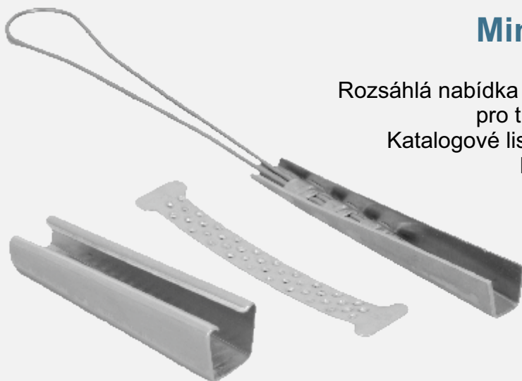
Kotva plochého závěsného kabelu
